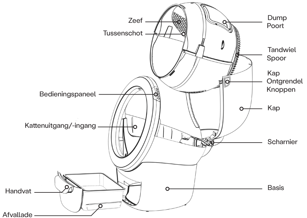
Explosietekening
