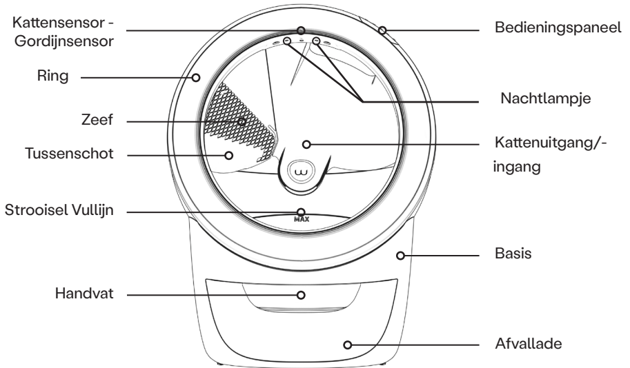
Vooraanzicht
